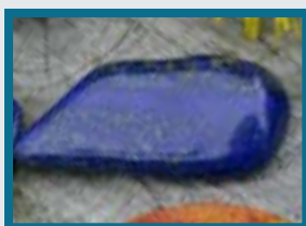
Лазурит с включениями Пирита
